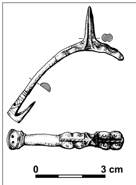
Ryc. 2. Słodkówko. Brązowa ostroga z zaczepami haczykowato zagiętymi do wnętrza. Rys. K. Zielińska
